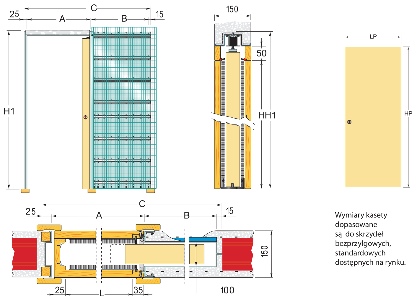
Wymiary kaset standardowych
