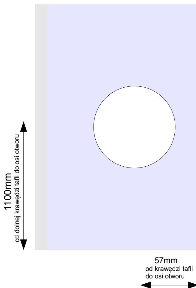
Otwór w tafli 47mm
