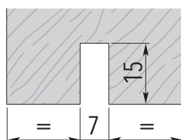
Wymiar frezu bez profilu aluminiowego
