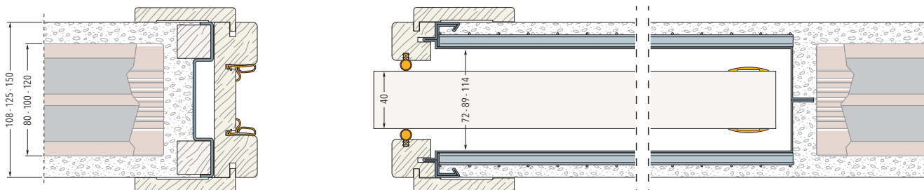
ECLISSE POJEDYNCZA - Całkowita grubość ściany 108/125/150 mm
