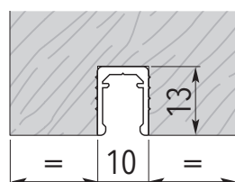
Wymiar frezu pod profil aluminiowy
