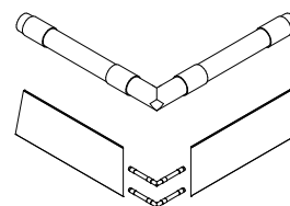
ŁĄCZNIK NAROŻNY ZEWNĘTRZNY
