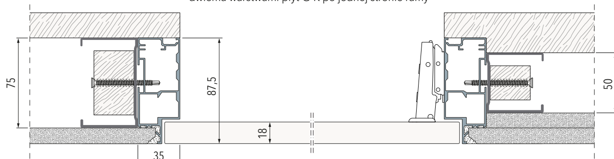
Ościeżnica do ścianki G-K z pojedynczym lub podwójnym opływowaniem
