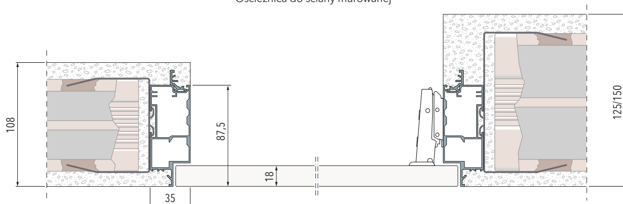
Ościeżnica do ściany murowanej
