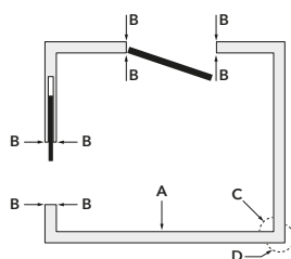
ŁĄCZNIK NAROŻNY WEWNĘTRZNY
