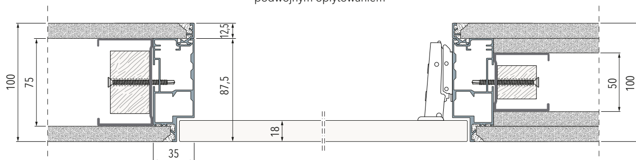
Ościeżnica do ścianki G-K z pojedynczym lub podwójnym opływowaniem montowana pomiędzy ścianami
