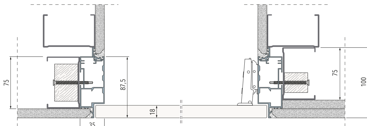
Ościeżnica do ścianki G-K z pojedynczym lub podwójnym opływowaniem montowana pomiędzy ścianami
