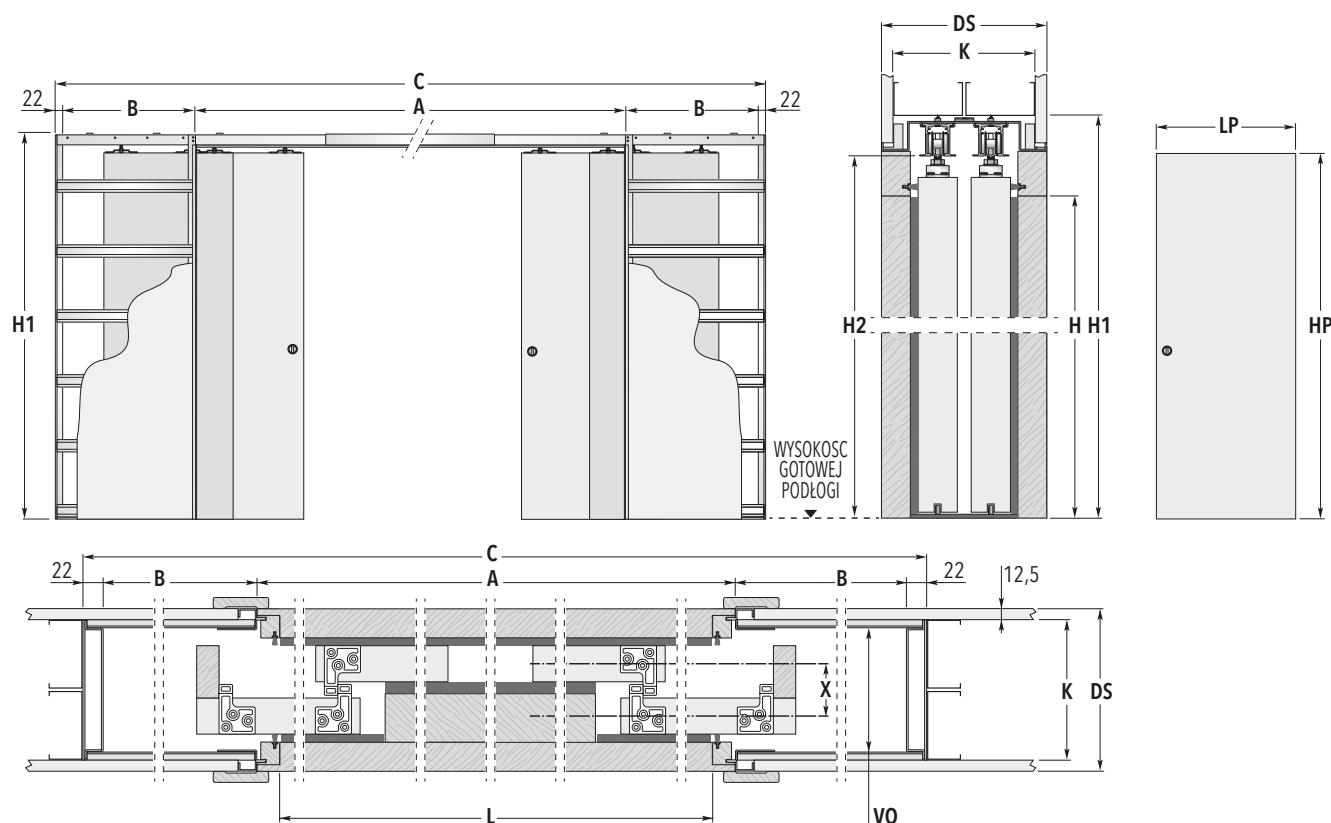
WYMIARY KASETY STANDARDOWEJ
