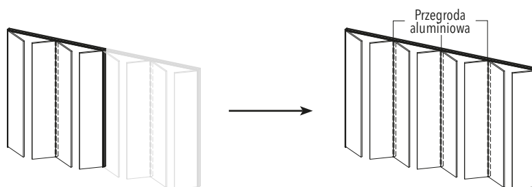
Ościeżnica 3-stronna zestaw do 8 skrzydeł
