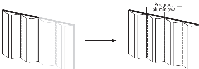
Ościeznica 3-stronna zestaw do 8 skrzydeł
